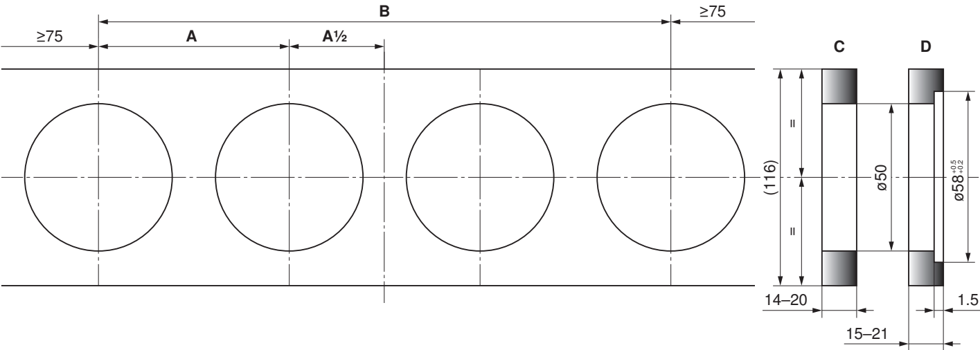
Masssskizze 4er-Set
