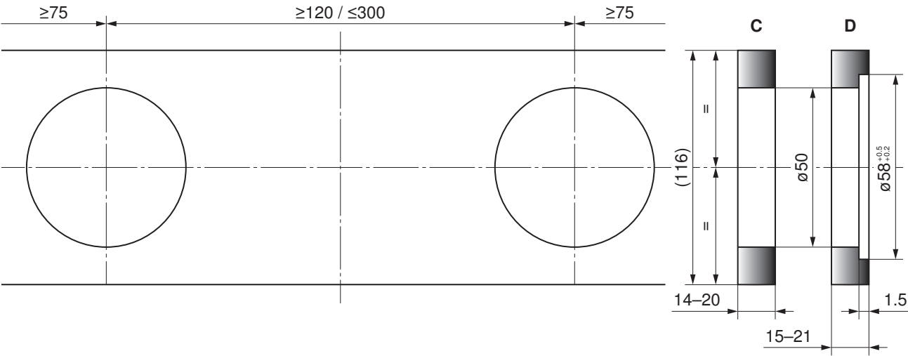
Masssskizze 4er-Set
